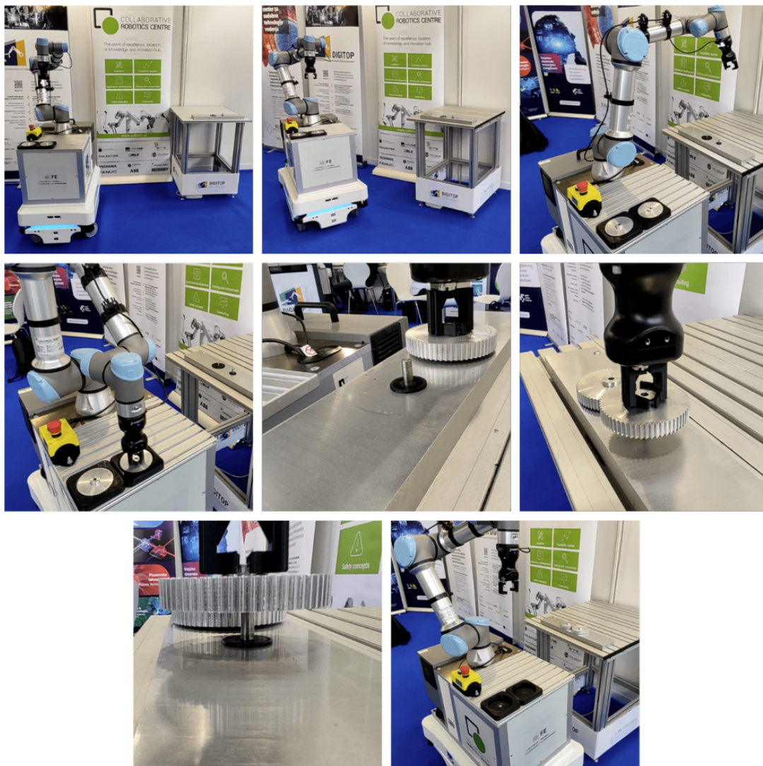
Slika 3: Izvedba aplikacije sestavljanja zobnikov (predstavljenjo na IFAM 2024 ( International trade for automation and mechatronics )).
