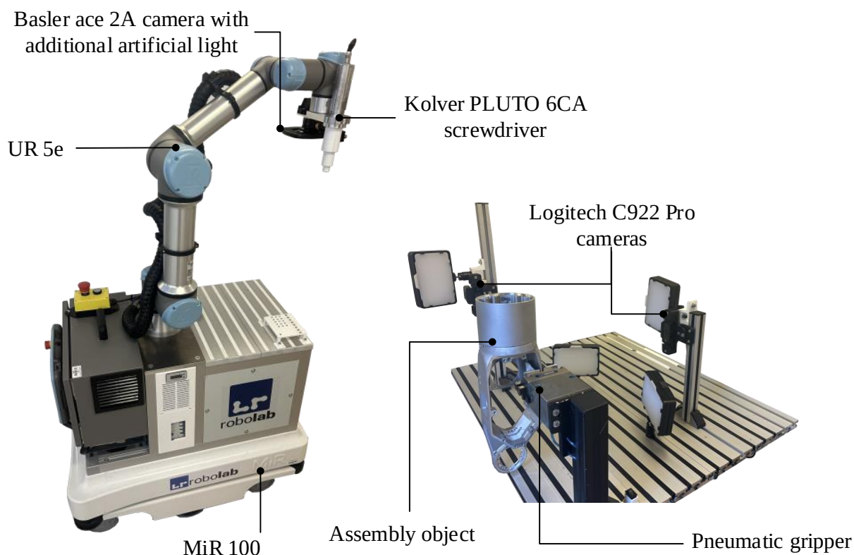
Slika 5: Pregled komponent: MiR100 + UR 5e z vijačnikom Kolver PLUTO 6CA, kamero Basler ace 2A in krožno LED; delovna postaja z dvema Logitech C922 Pro, LED paneloma in pnevmatskim prijemalom.
