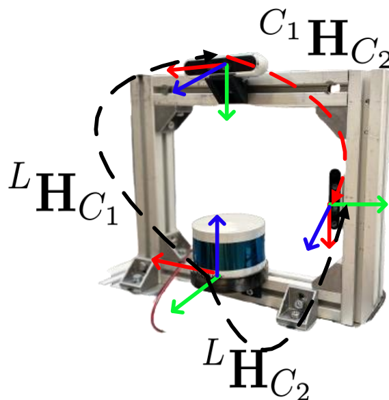
Slika 12: Primer multimodalnega senzorskega sistema, ki vsebuje 3D LIDAR in 2 globliski kameri. Na sliki so označeni, še transformaciji med senzorji, ki jih probamo določiti s pomočjo metode ekstrinzične kalibracije, ki jo razvijamo.
