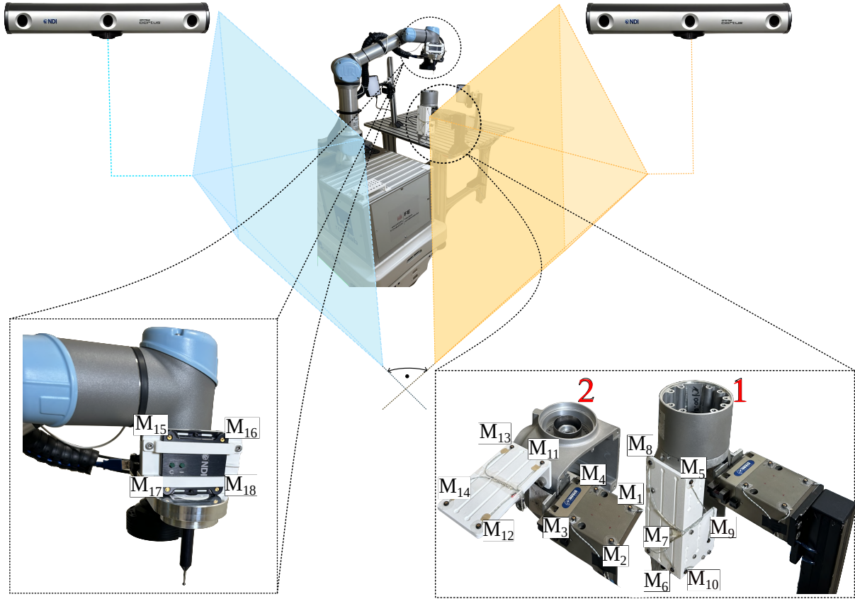
Slika 10: Merilni sestav z OptoTrak Certus in označitvijo markerjev na delovni postaji, objektih in tipalu.
