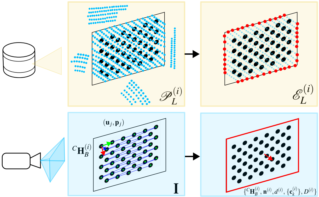
Slika 13: Podatki pri posameznemu zajemu uporabljeni za optimizacijo. Za vsak sinhroniziran par najprej (zgoraj) iz oblaka LiDAR izluščimo planarno tablo in robne vzorce, nato pa (spodaj) iz slike zaznamo mrežo krogov in ocenimo pozo table v koordinatnem sistemu kamere.
