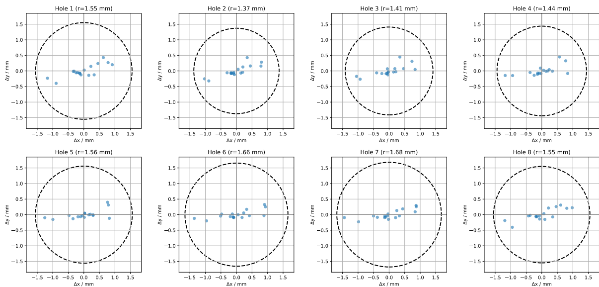
Slika 11: Ponovljivost translacijskega pozicioniranja vijačnika v ravnini xy za luknje 1–8.
