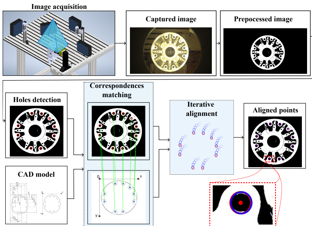
Slika 8: Detekcija lukenj in CAD-poravnava: detekcija krogov → vzpostavljanje ujemanj → iterativna afina poravnava → metrična pretvorba.
