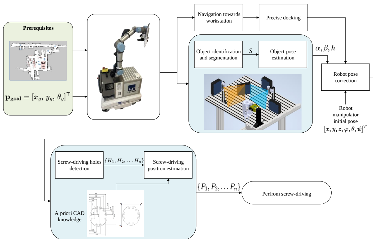
Slika 6: Potek pristopa: navigacija → precizno pozicioniranje v končni legi → (vzporedno) identifikacija, segmentacija in ocena nagiba/višine → korekcija lege → zajem slike s kamero na vrhu robota → detekcija lukenj in CAD-poravnava → vijačenje.
