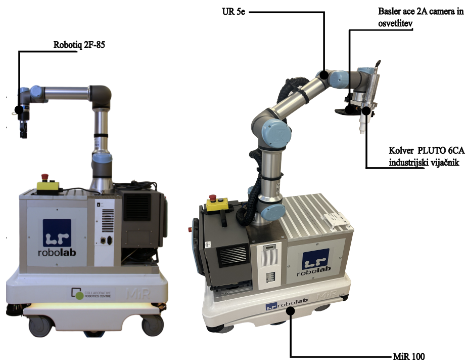
Slika 2: Sestavni deli modularnega mobilnega sodelujočega robotskega sistema.
