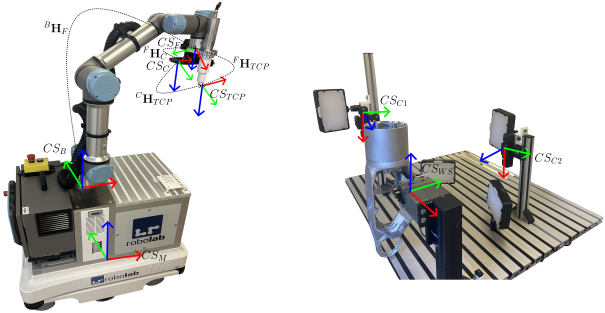
Slika 9: Prikaz vseh relevantnih koordinatnih sistemov (CS) in prostorskih transformacij ( \mathbf{H} ), ki se uporabljajo pri kalibraciji sistema in izvajanju nalog. Koordinatni sistemi so določeni na naslednji način: CS_B predstavlja osnovni koordinatni sistem robotskega manipulatorja, CS_M osnovni koordinatni sistem mobilne platforme, CS_F koordinatni sistem robotske prirobnice, CS_C koordinatni sistem kamere, nameščene na robotu, CS_{TCP} koordinatni sistem orodja na delovni točki (TCP) vijačnika, CS_{WS} lokalni koordinatni sistem delovne postaje, ter CS_{C1} in CS_{C2} koordinatna sistema kamer, nameščenih na delovni postaji. Pripadajoče transformacije so opredeljene na naslednji način: {}^F\mathbf{H}_C predstavlja transformacijo med koordinatnima sistemoma robotske prirobnice in kamere, {}^F\mathbf{H}_{TCP} transformacijo med prirobnico in orodjem (TCP), ter {}^B\mathbf{H}_F transformacijo med osnovo robota in njegovo prirobnico. Dodatne transformacije so definirane po analogiji, kjer je to ustrezno.
