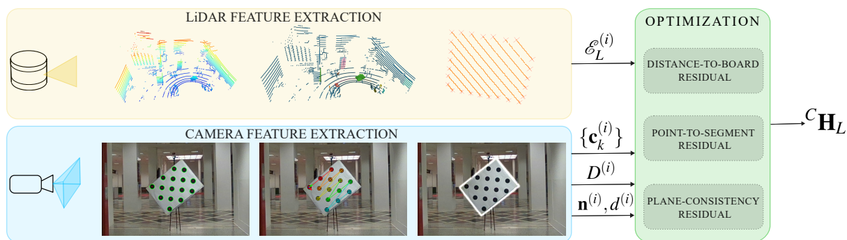
Slika 14: Pregled predlaganega kalibracijskega postopka LiDAR–kamera. (Zgoraj) iz oblaka točk z gručenjem in oblikovnim filtriranjem izluščimo planarno tablo in robne točke. (Spodaj) v sliki zaznamo asimetrično mrežo krogov in ocenimo pozo table. (Desno) optimizator združuje slikovne in prostorske geometrijske omejitve skozi več pogledov ter vrne transformacijo \text{LiDAR} \rightarrow \text{kamera} .
