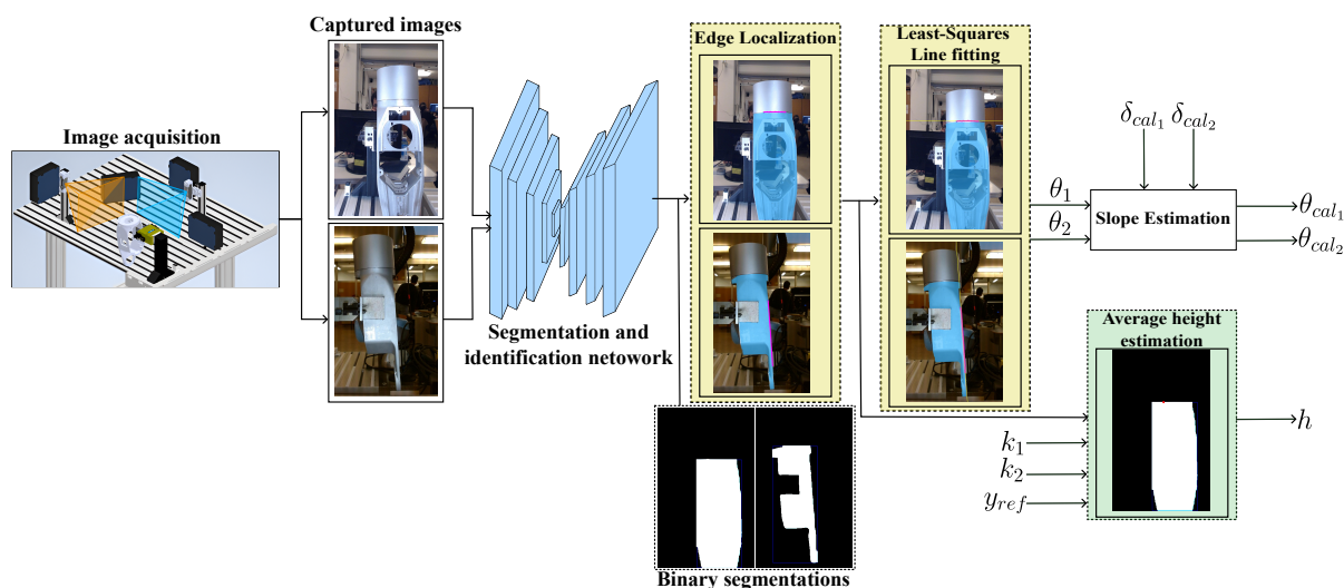
Slika 7: Potek algoritma za identifikacijo objekta in ocena njego lege v prostoru..
